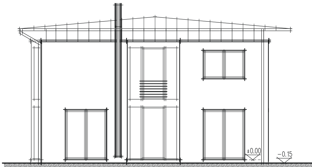
Rückansicht Stadtvilla
