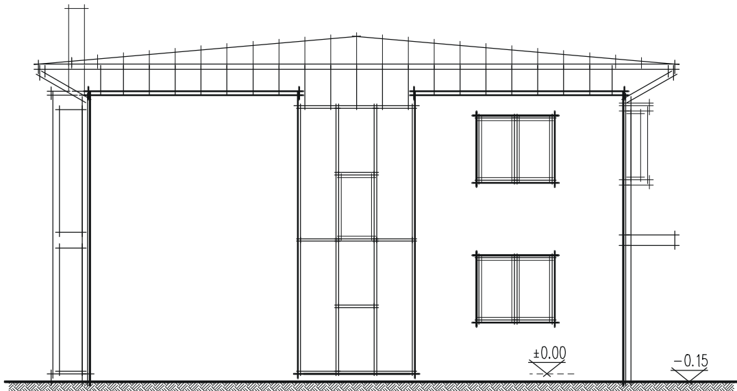
Seitenansicht Stadtvilla
